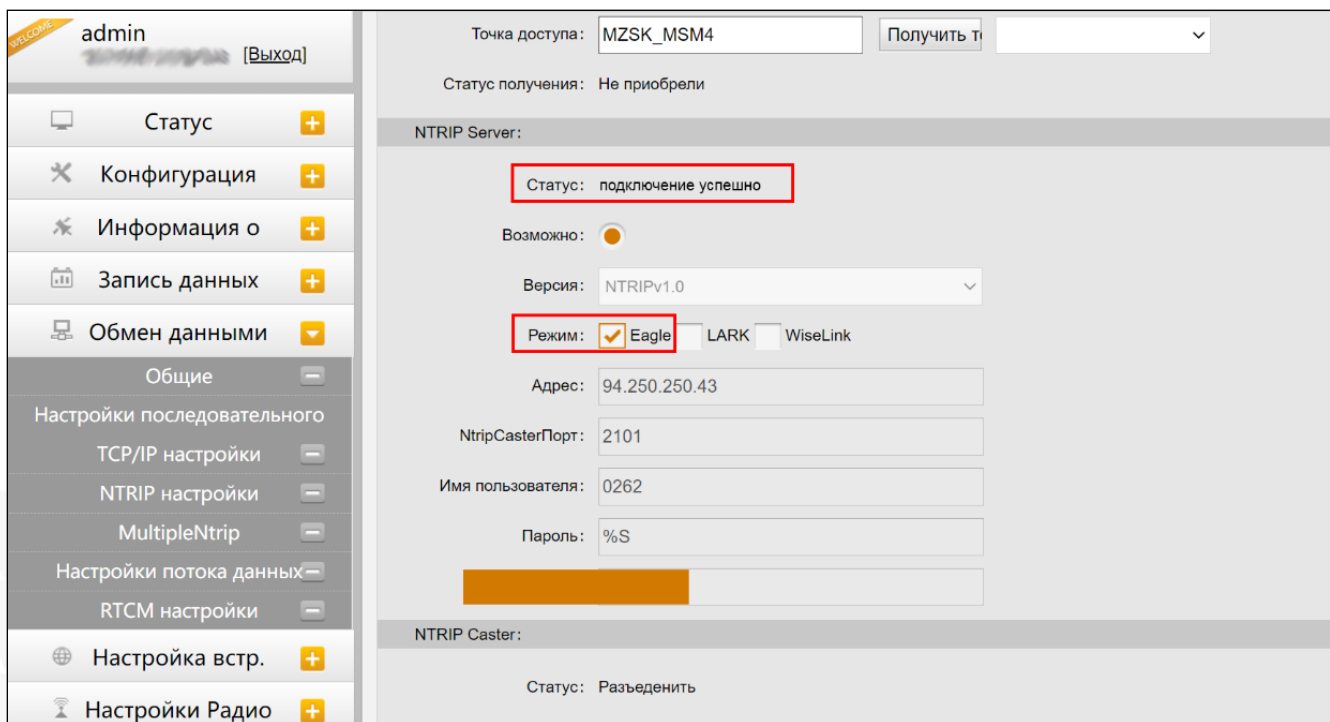
Веб-интерфейс, вкладка Обмен данными-Ntrip настройки-Ntrip server
