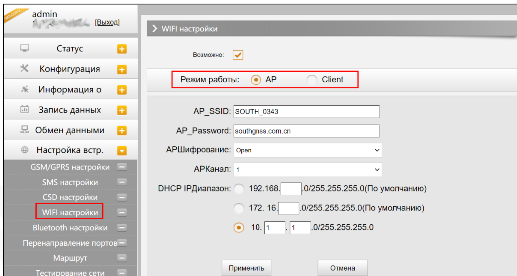
Веб-интерфейс, вкладка Настройки вст. GSM-WIFI настройки
