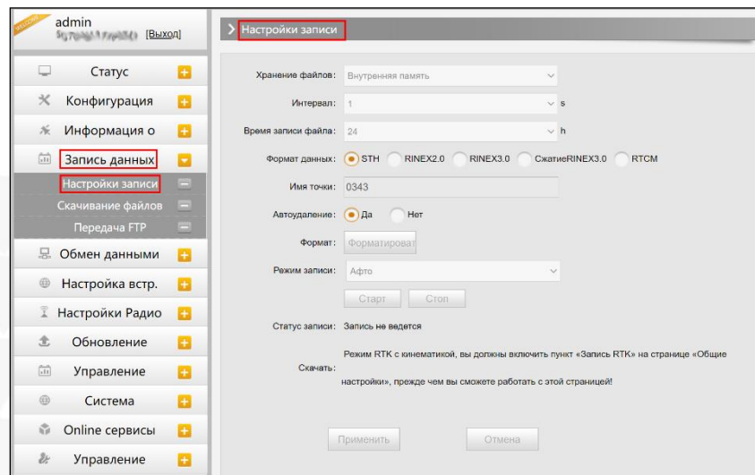
Веб-интерфейс, вкладка Запись данных-Настройки записи
