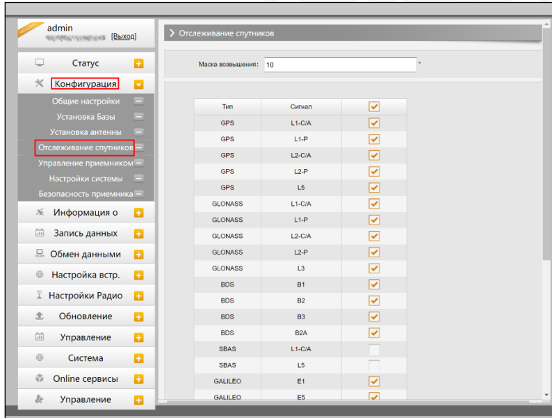
Веб-интерфейс, вкладка Конфигурация-Отслеживание спутников
