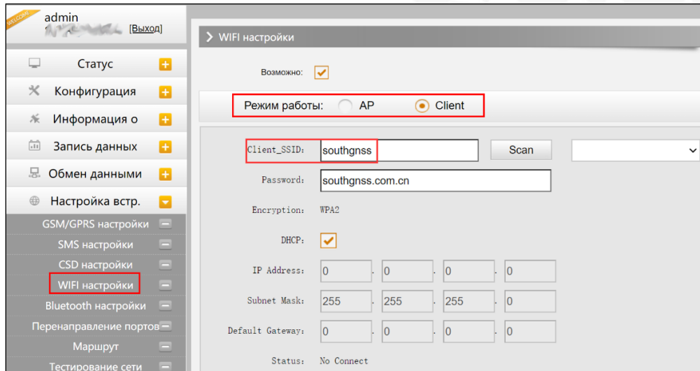
Веб-интерфейс, вкладка Настройки втр. GSM-WIFI настройки-Client
